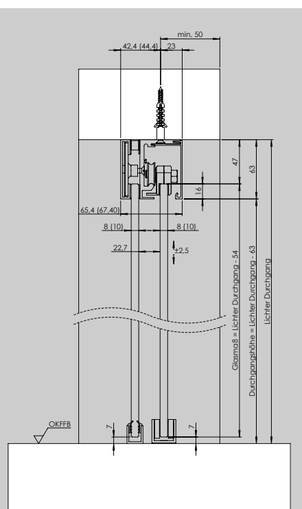
PLNEO 120, DECKENMONTAGE FÜR GLASANLAGEN CEILING MOUNTING FOR GLASS DOOR SYSTEM
