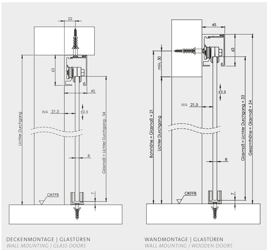
PLANEO 120 DECKENMONTAGE FÜR RAUMHOHE LÖSUNGEN CEILING MOUNTING FOR FLOOR-TO-CEILING SOLUTIONS
